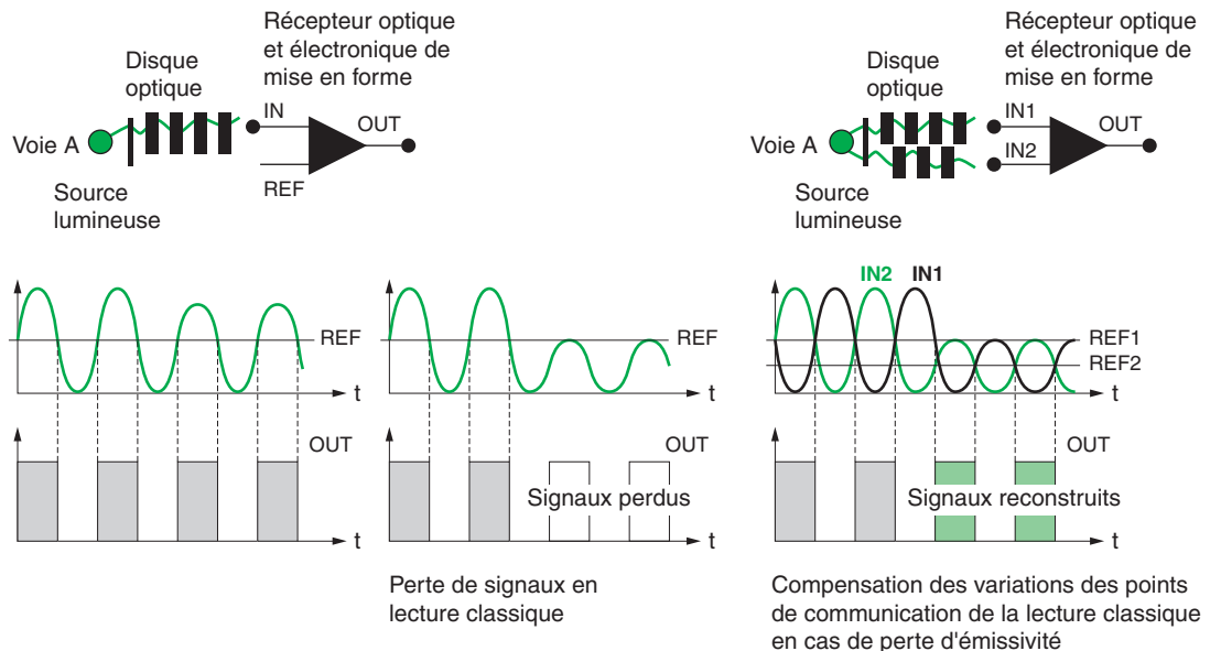
Fig. 51 : principe pour reconstruire un signal émis.
