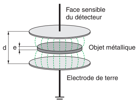
Fig. 10 : présentation d'un objet conducteur sur un détecteur capacitif.
