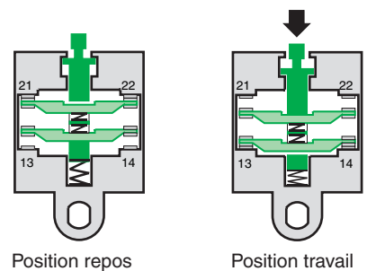
Fig. 4 : exemple d'un contact à action dépendante.
