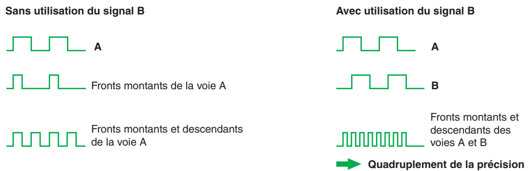
Fig. 49 : principe pour quadrupler la précision d'exploitation.
