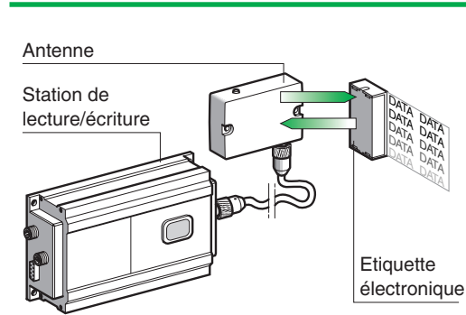
Fig. 29 : présentation des éléments d'un système RFID (Système Inductel de Telemecanique).
