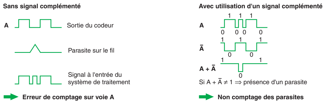
Fig. 50 : signaux complémentés permettant de différencier les impulsions et d'éviter ainsi la prise en compte des impulsions parasites.
