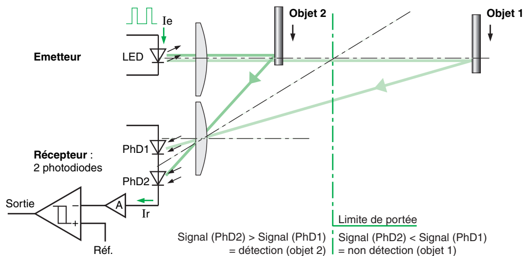
Fig. 20 : principe de la détection photoélectrique à réflexion directe avec suppression de l'arrière plan.
